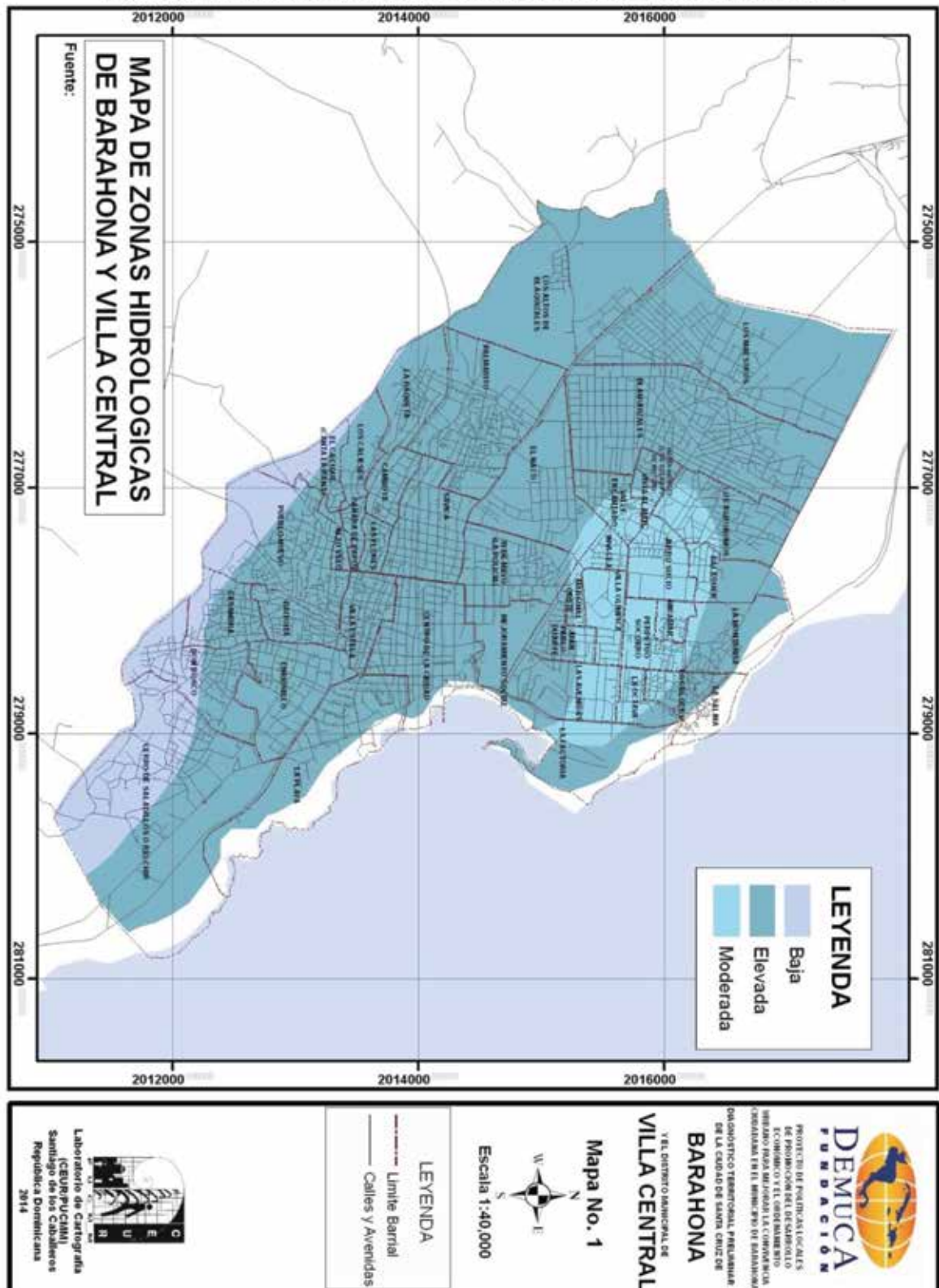
FIGURA 10. MAPA DE ZONAS HIDROLÓGICAS Y DE PRODUCTIVIDAD DE ACUIFEROS
