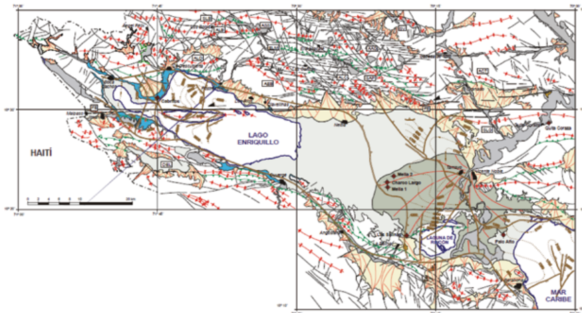
FIGURA 4. ESQUEMA ESTRUCTURAL DEL AREA DE ESTUDIO. SIERRA DE NEIBA, VERTIENTE NORTE SIERRA DE BAHORUCO Y CUENCA DE ENRIQUILLO.
