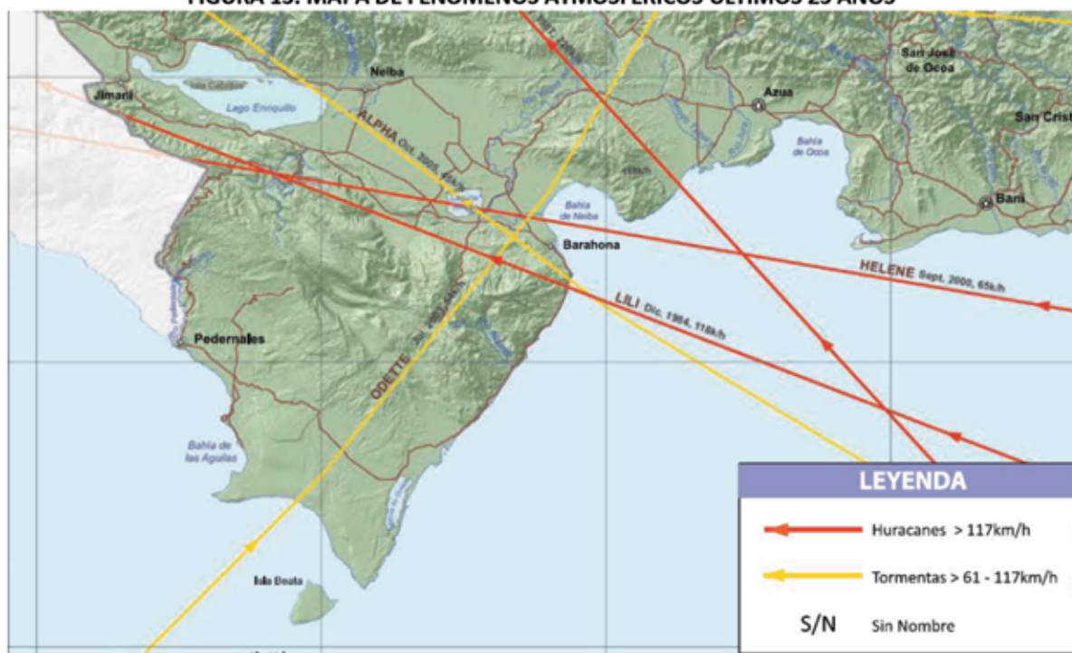
FIGURA 13. MAPA DE FENOMENOS ATMOSFERICOS ULTIMOS 25 AÑOS
