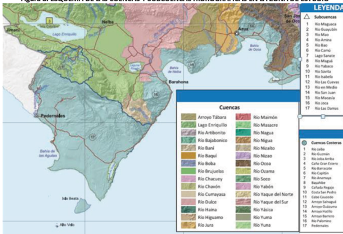
Figura 8. ESQUEMA DE LAS CUENCAS Y SUBCUENCAS HIDROGRAFICAS EN LA ZONA DE ESTUDIO
